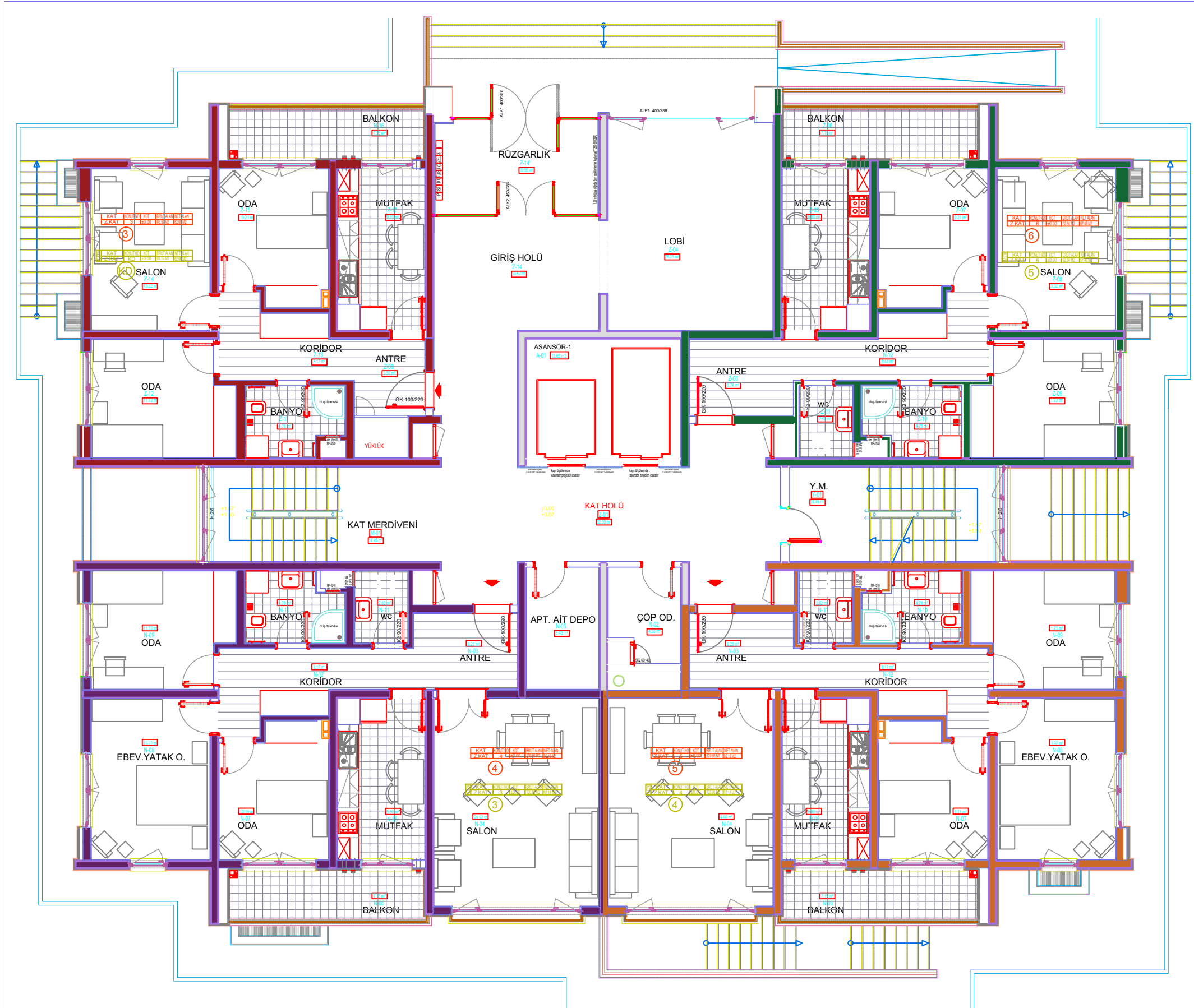
ANKARA SINCAN SARAYCIK MAHALLESİ G.Ö.B. KENTSEL DÖNÜŞÜM PROJESİ SC2 TİP BLOK ZEMİN KAT PLANI
